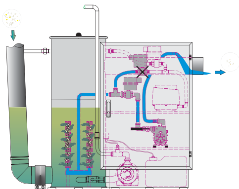
Funktionsprinzipien von Haustechnikanlagen werden in Seminaren veranschaulicht
