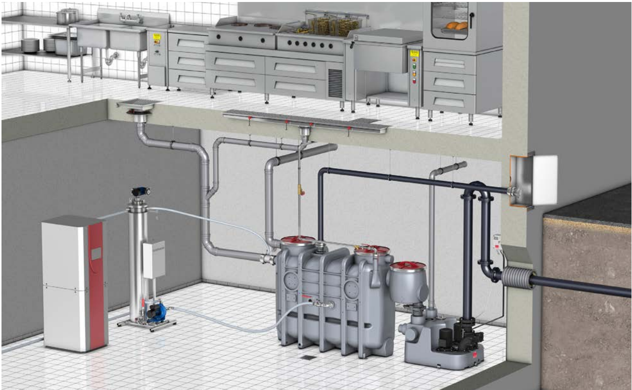
Wärmepumpe mit Wärmetauscher, angeschlossen an einen Fettabscheider (mit Probenahme und Hebeanlage) mit entsprechender Verrohrung an die Entwässerungsgegenstände der Großküche.
