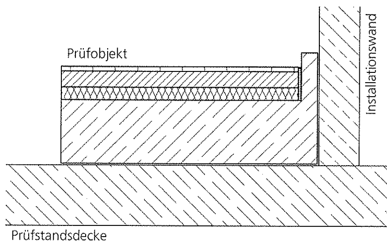
Bild 11: Schnittzeichnung des Prüfaufbaus im Installationsprüfstand P12 des IBP (ohne Maßstab).
