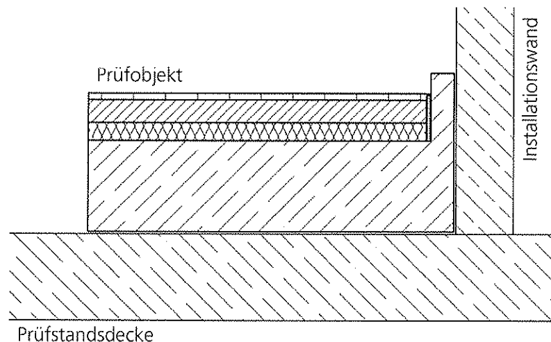
Bild 11: Schnittzeichnung des Prüfaufbaus im Installationsprüfstand P12 des IBP (ohne Maßstab).
